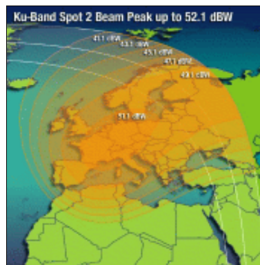
Spot 2-nyaláb
