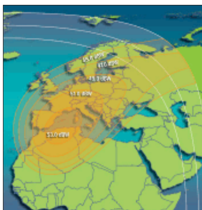
Spot 1-nyaláb
