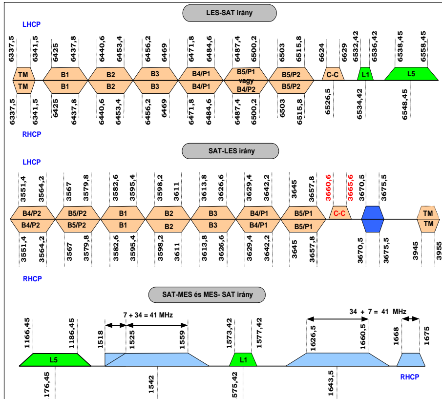
5. ábra. Az Inmarsat-4 frekvenciasáv kiosztása
