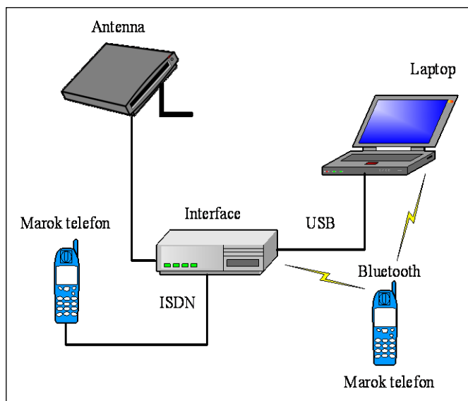
8. ábra. Perifériák csatlakozása a terminálhoz
