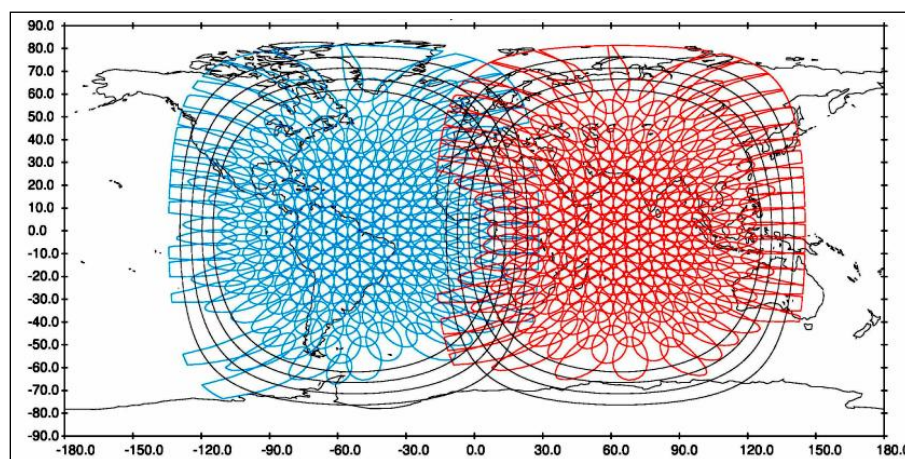
4. ábra. A kis nyílásszögű beamek (két műhold)
