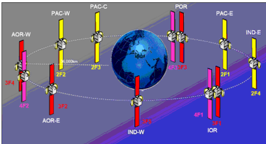
2. ábra. Az Inmarsat rendszer műholdjainak elhelyezkedése
