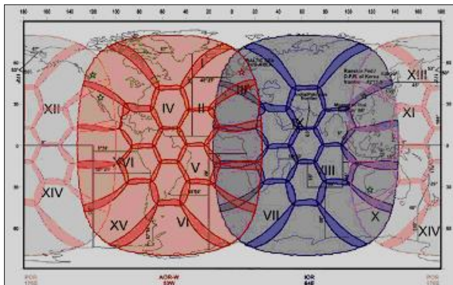
3. ábra. A nagy nyílásszögű beamek
