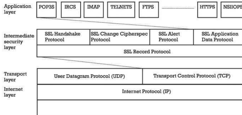
5. ábra. Az SSL felépítése. A rekord (Record), a kapcsolat-felépítés (Handshake), a rejtjelező beállításváltója (Cipherspec Change) és a riasztó eseményt kezelő/jelző (Alert) összetevő protokollok elhelyezkedése, valamint a rájuk épülő, biztonságosnak tekintett alkalmazások
