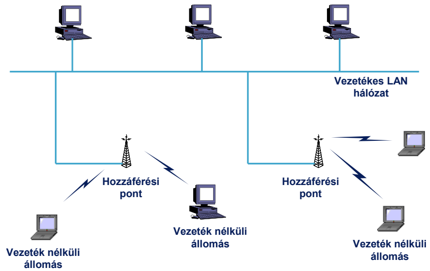
2. ábra. WLAN-hálózat a vezetékes LAN-hálózathoz illesztve
