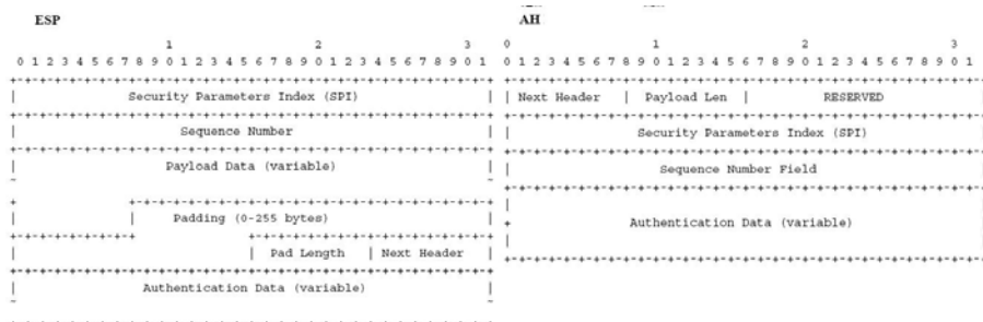
9. ábra. Az ESP (Encapsulated Security Payload) és AH (Authentication Header) protokollok bitmezői
