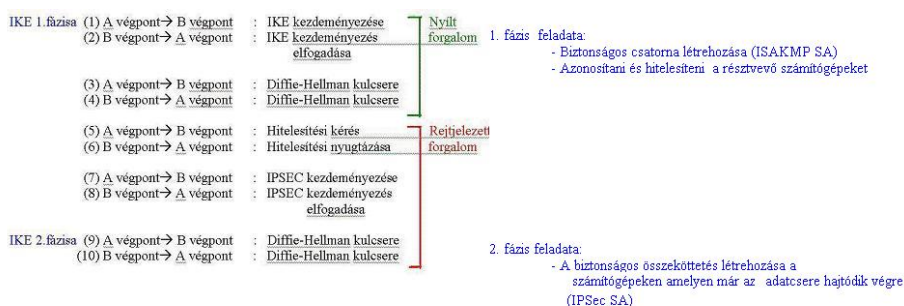
10. ábra. Az IKE két fázisának elvi lépéseinek modellje, minimum 10 lépésben
