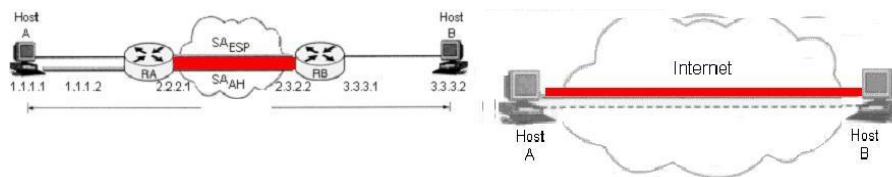
12. ábra. IPsec-alagút módot alkalmazó, internet-részhálózathoz és belső hálózathoz felépülő modellhálózat, és egy minimális hálózat a szállítási mód bemutatására
