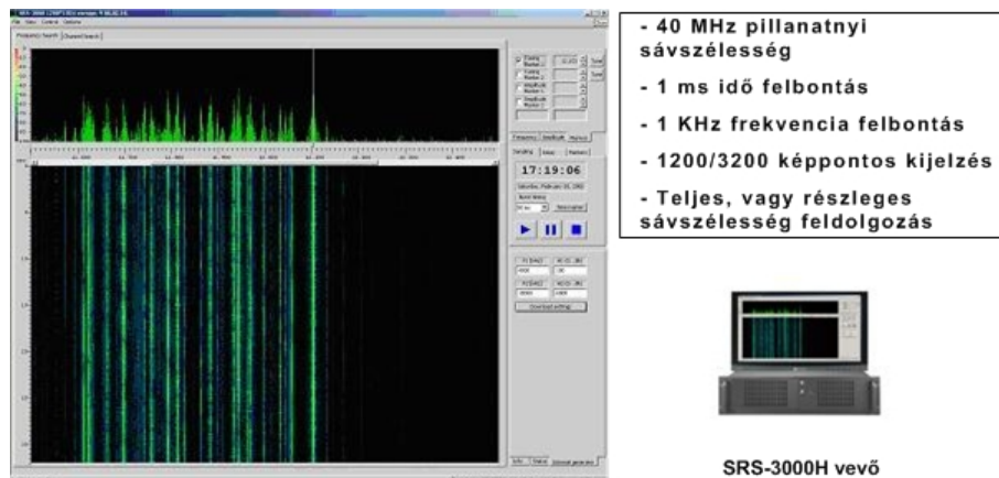
14. ábra. Széles sávú panoráma-vevőkészülék
