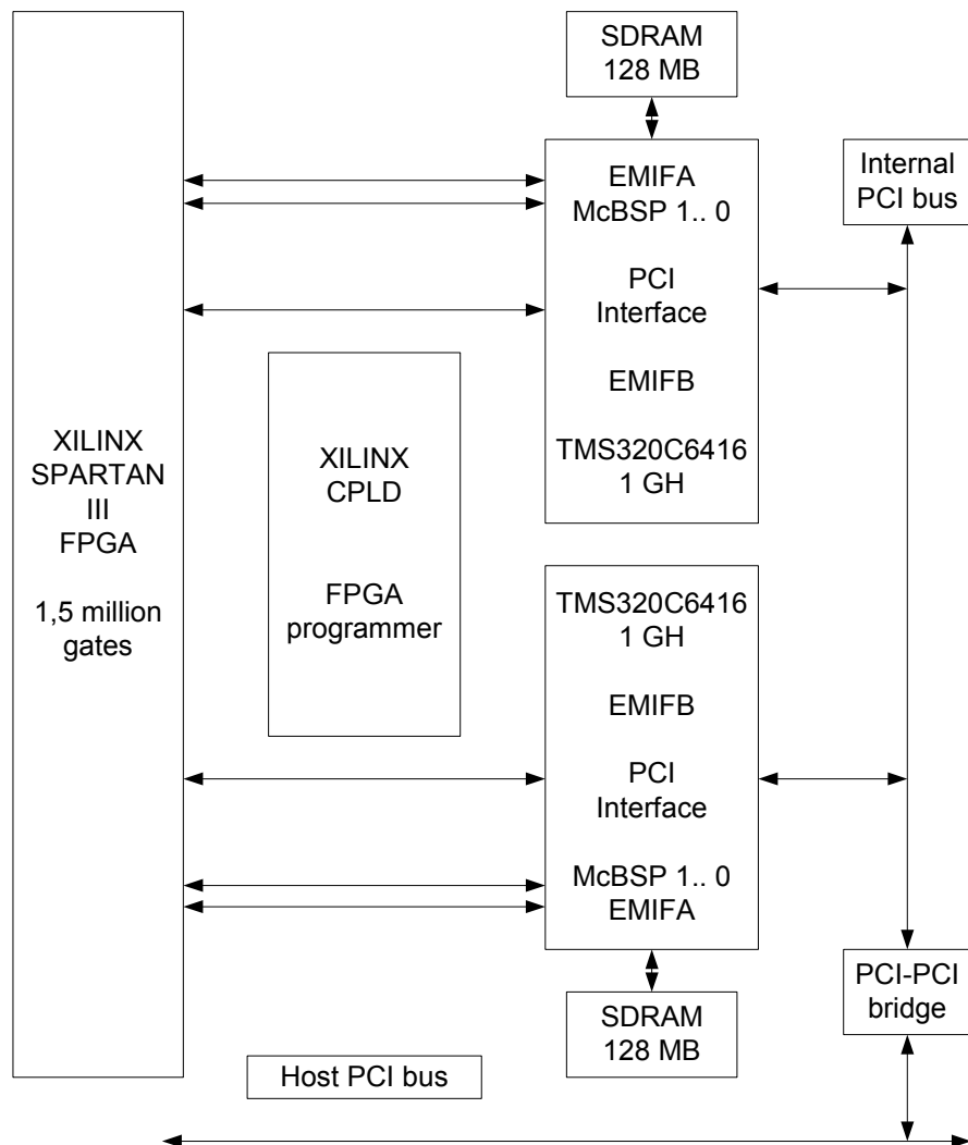
1. ábra. A PCDSP6 kártyacsalád közös magja
