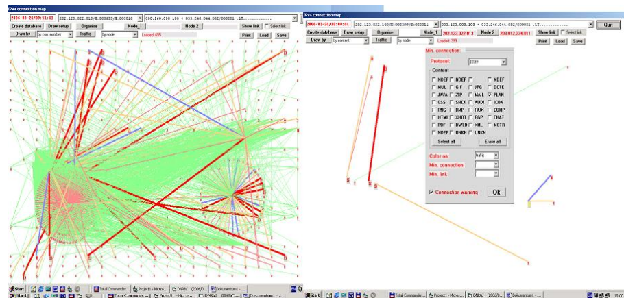
3. ábra. Balra az adatáramlás és a vezérlés együttese, míg jobbra a vezérlés és a hozzá kapcsolódó protokoll-szűrés eredménye egy adott célhálózatra, illetve a riasztás beállítása egy várt kapcsolat megjelenésének észlelésére
