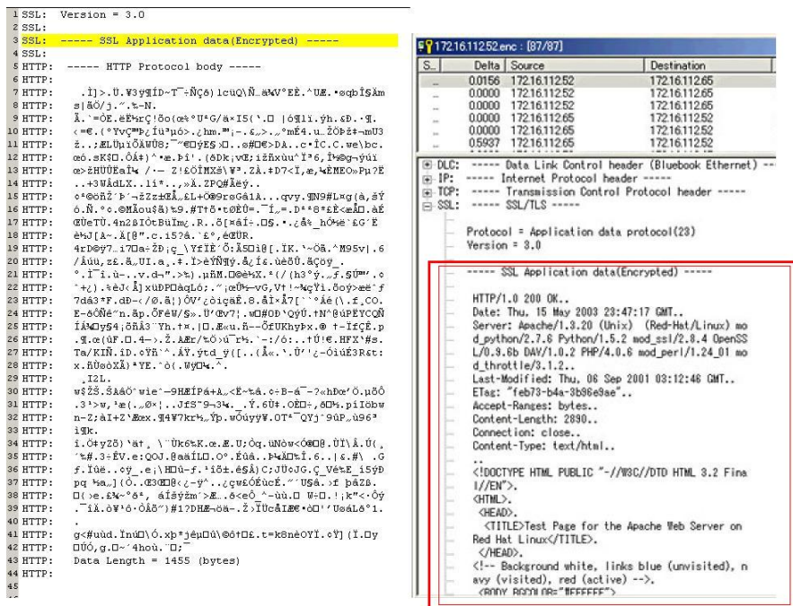
22. ábra. Az SSL/VPN csomag kibontása
