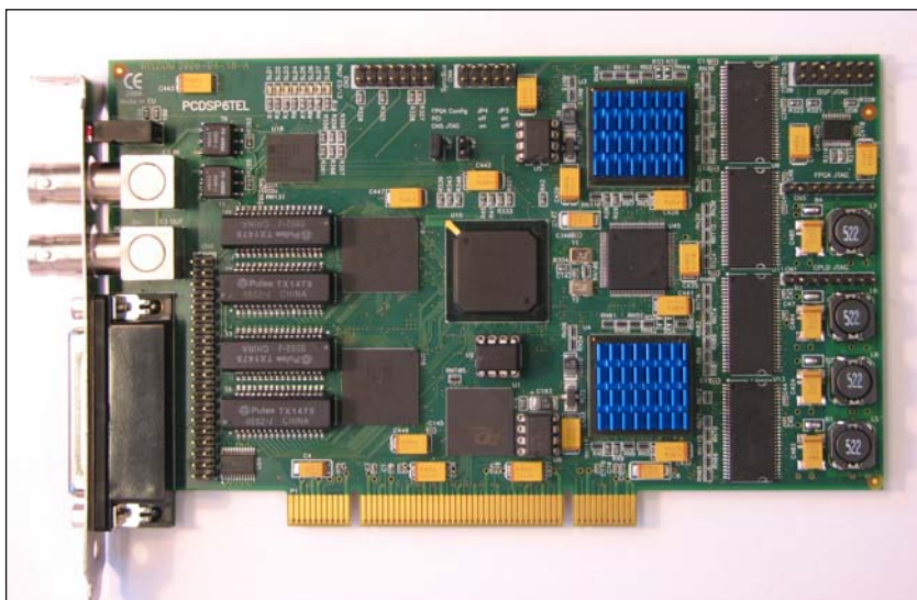
5. ábra. A PCDSP6TEL telekommunikációs alkalmazásokra specializált jelfeldolgozó kártya
