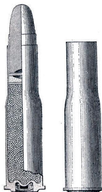
62. 1877 M Werndl lőszer
