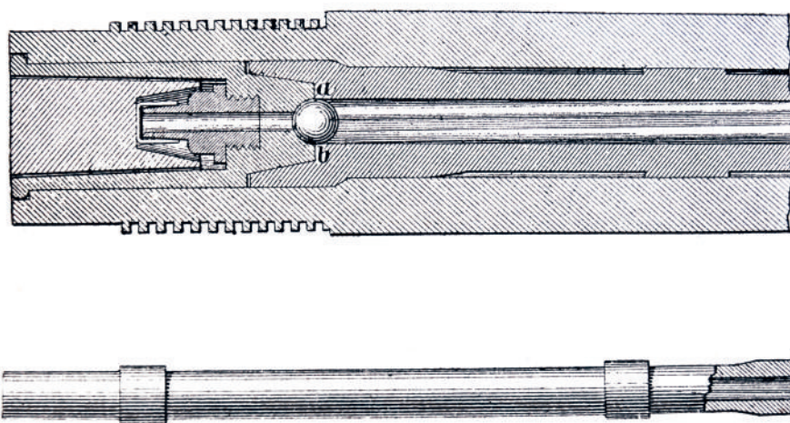
82. Werndl szobai céllövő betétcső
