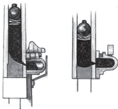
5. Önfelporzó és kónikus gyúlyukkal rendelkező kovás csőfar
