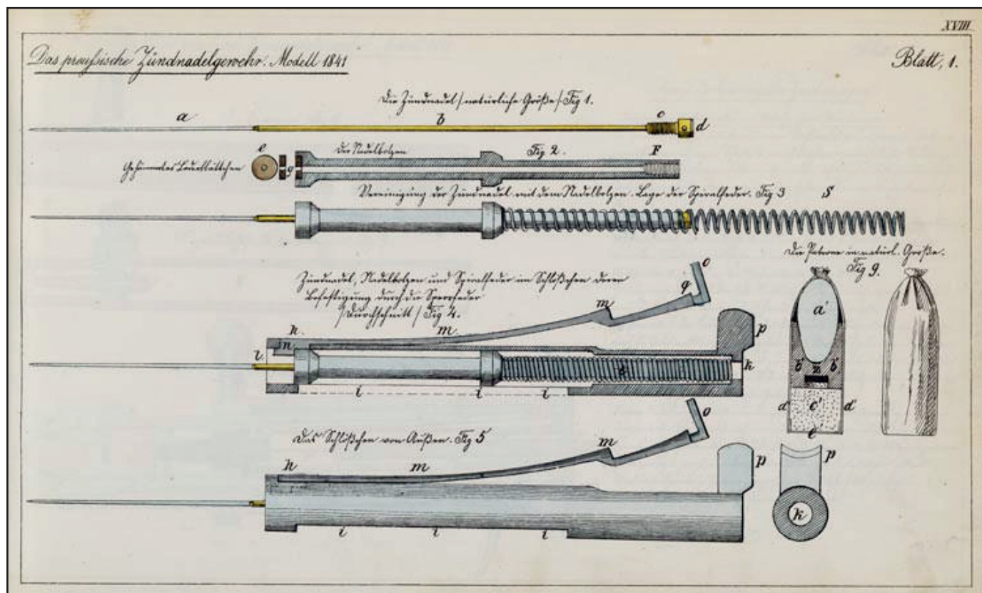
35. A Dreyse puska zárszerkezete és tölténye
