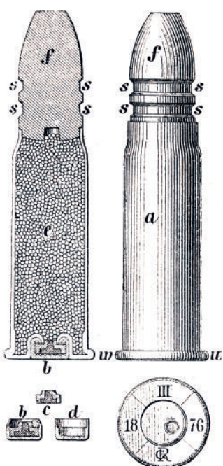
61. 1867 M Werndl lőszer
