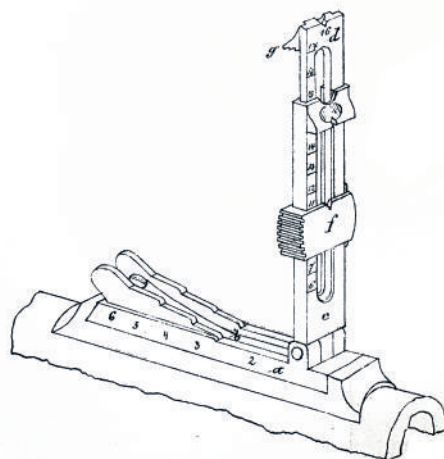
68. Werndl 1877 M nézőke
