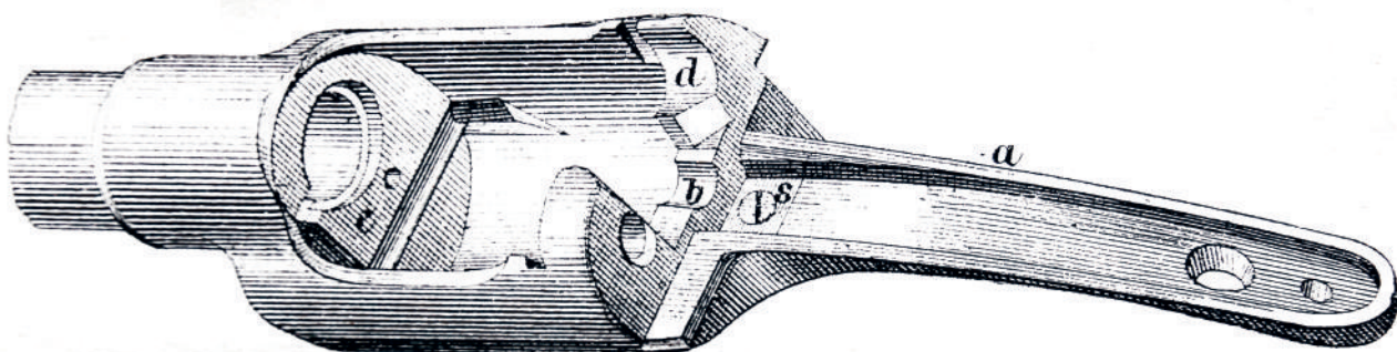
58. 1867 M Werndl tokszerkezet
