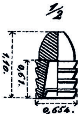
10. Francia M 1853 Minié löv.
