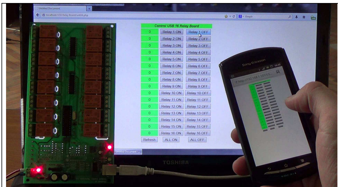
56. ábra – Vezérelhető USB relék 90
